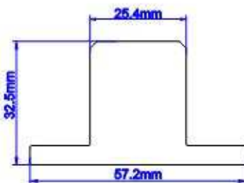
Chamfer T Post (Deco)
